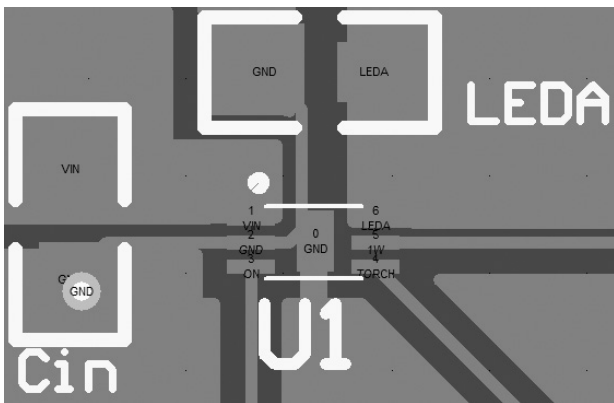
图 6. U1DFN-1.5x2-6L 的 PCB 布线图
