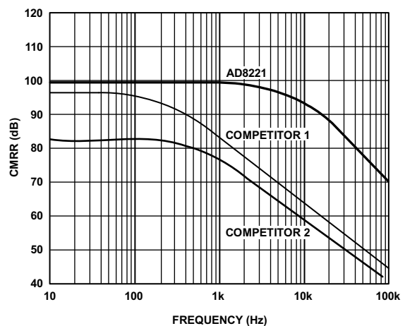
图2. 典型CMRR与频率的关系( G = 1 )
