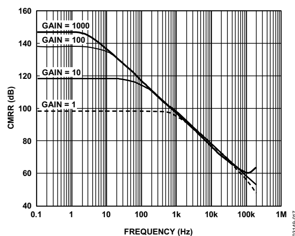
图17. CMRR与频率的关系(RTI, 1 kΩ非均衡信号源)
