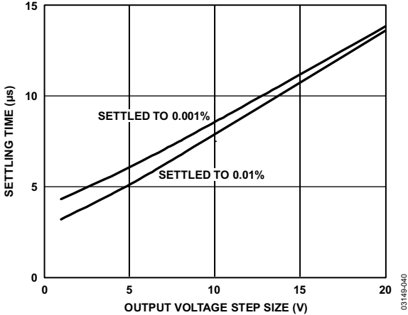
图40. 建立时间与步进大小的关系( G = 1 )
