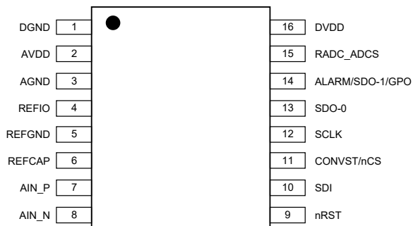
TSSOP-16
