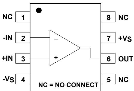
SOIC-8
