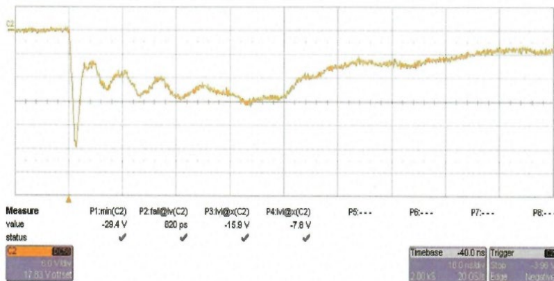
Negative 8kV:
