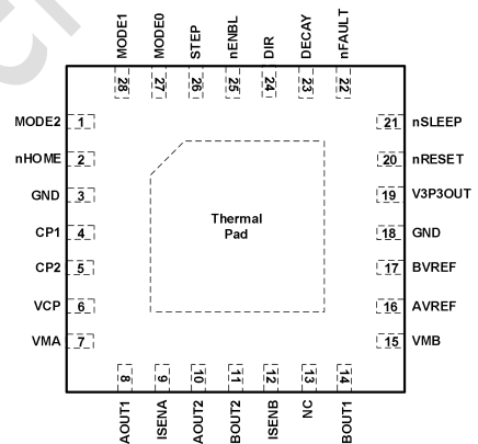
QFN5*5-28(Top view) TMI8420Q
