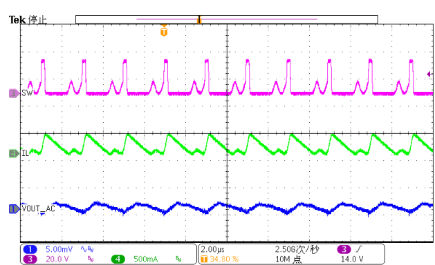
Figure 21. Output Ripple (Iload=100mA)
