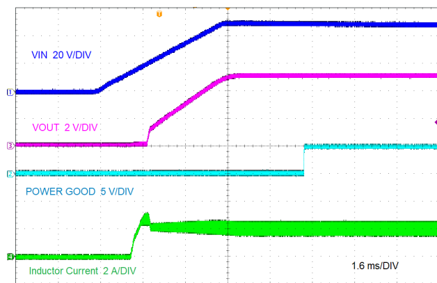
LMR38020-Q1 V_{OUT} = 5\text{ V} 400 kHz
